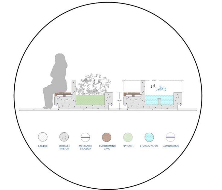
ΚΑΤΑΣΚΕΥΑΣΤΙΚΗ ΛΕΠΤΟΜΕΡΕΙΑ ΠΑΓΚΟΥ
